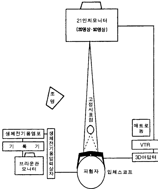
그림 1. 2D영상과 3D영상 관찰시의 실험장치도(실험1)
